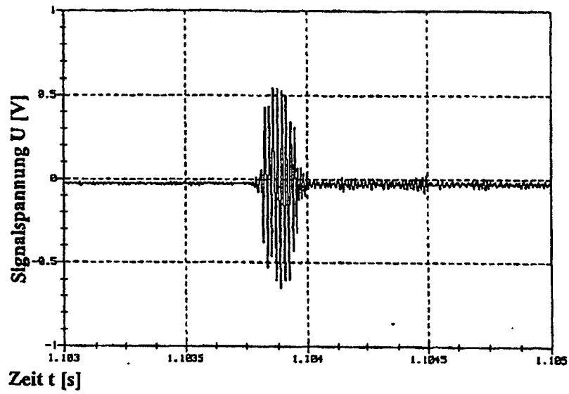
Kontinuierliche Schallemission infolge Gelenkreibung
